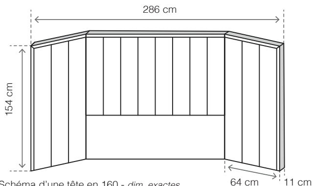
Schéma d'une tête en 160 - dim. exactes
