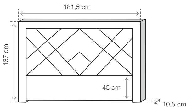
Schéma d'une tête en 160 - dim. exactes
